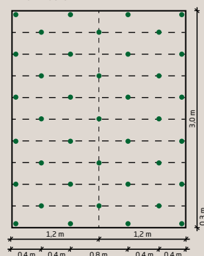
Böschung > 1:1 4-6 Pflöcke/m 2
