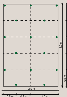
Böschung < 1:1 2-3 Pflöcke/m 2
