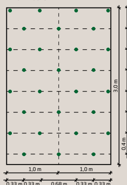
Böschung > 1:1 4-6 Pflöcke/m 2
